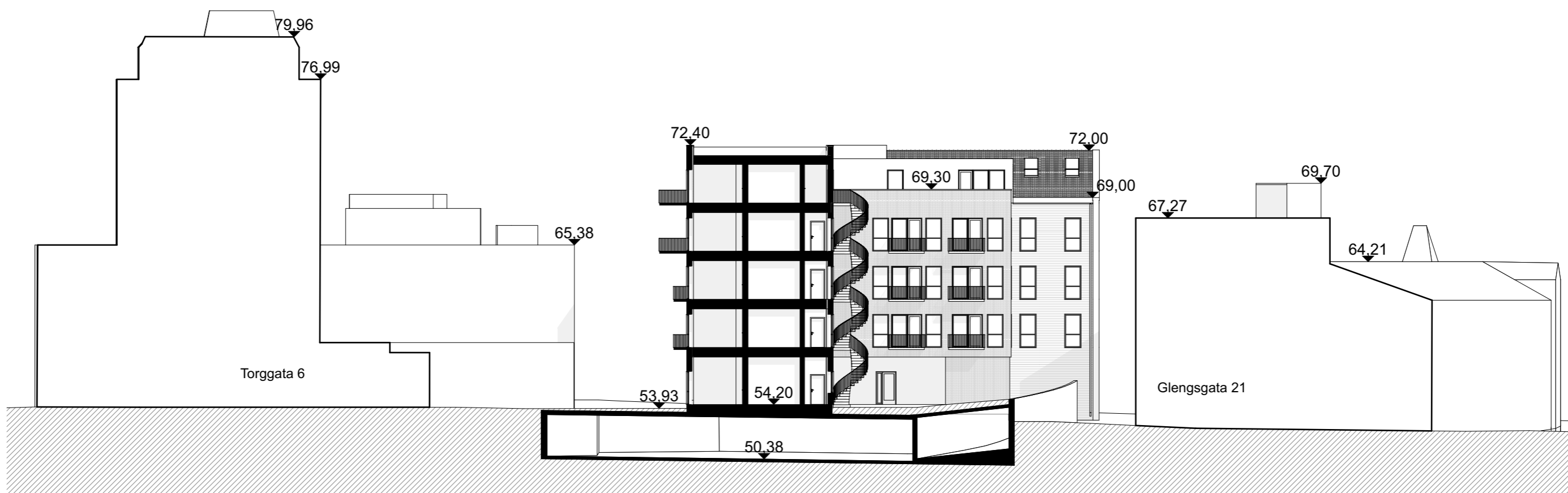
Snitt A-A 1:300
