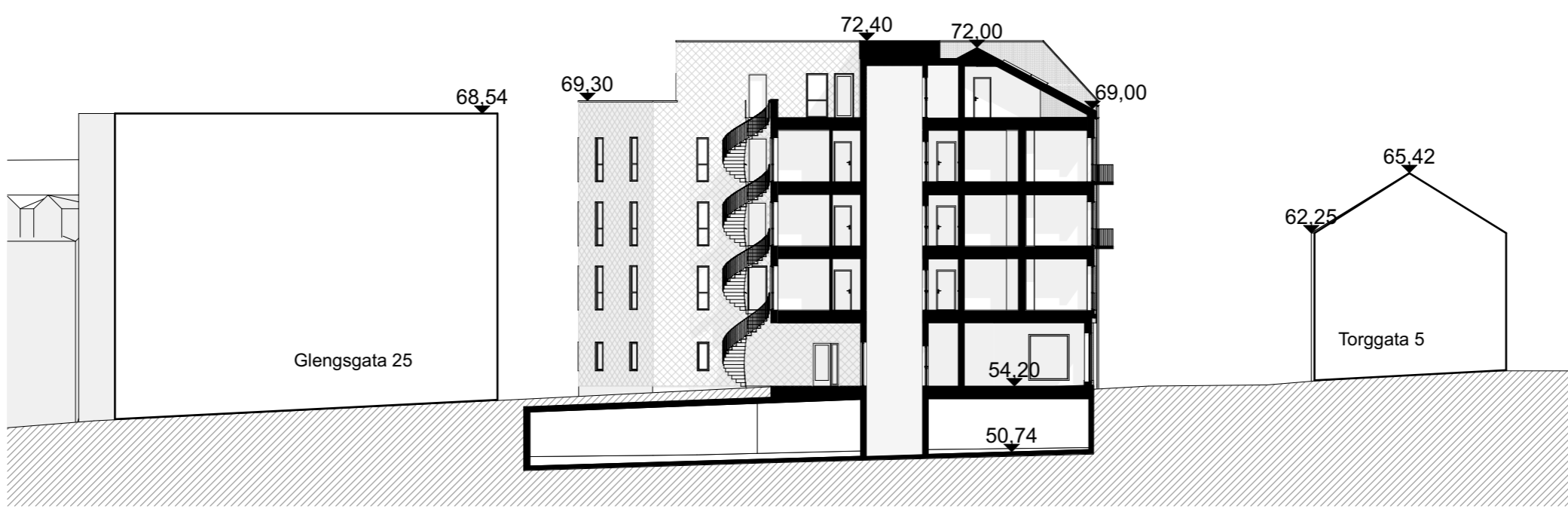
Snitt B-B 1:300
